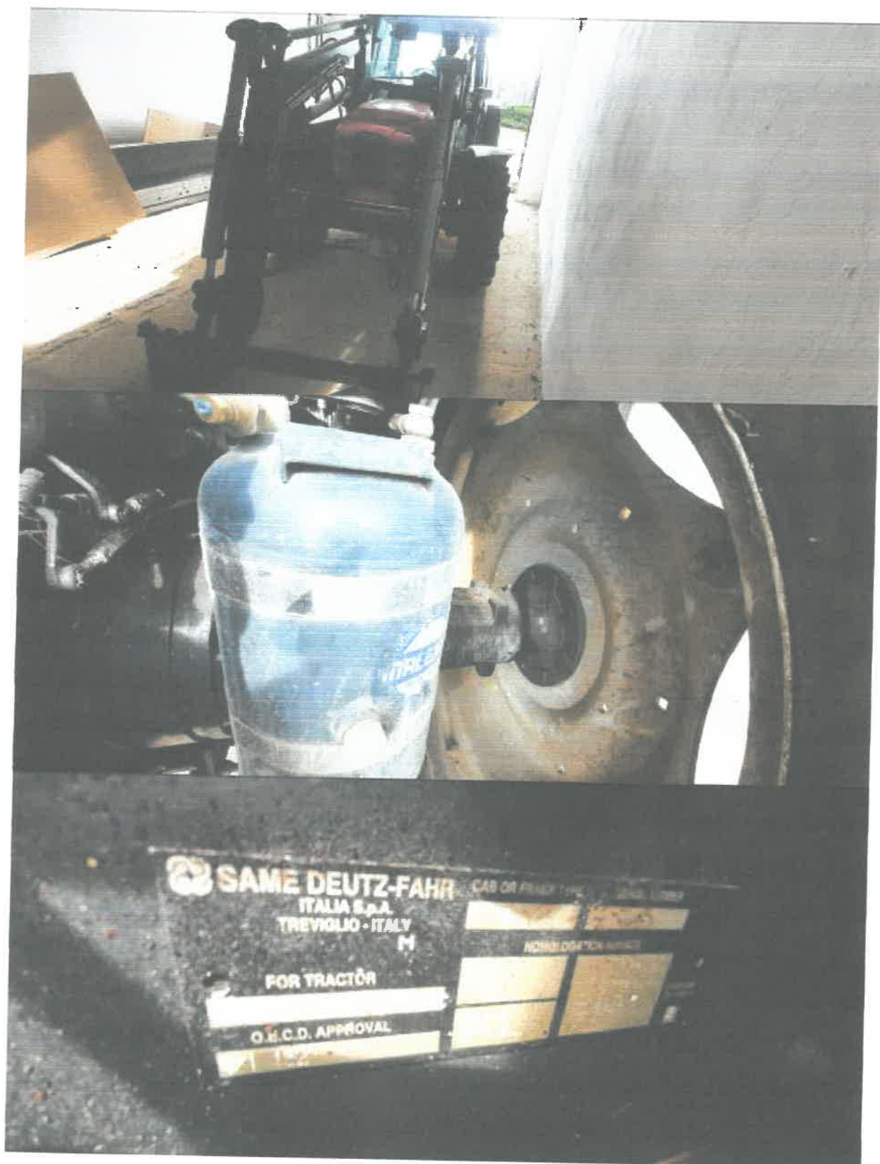
Ciągnik rolniczy – marki SAME, typ: 10S, rok produkcji: 2010
